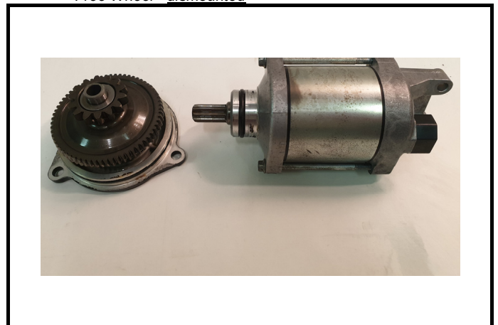
C16-2) Roue libre - déposée Free Wheel - dismounted
